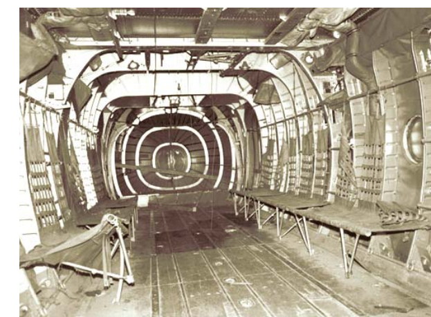
➤ Το εσωτερικό ενός Noratlas βλέποντας προς τα πίσω
